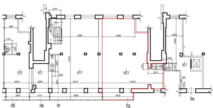
1 ЭТАЖ
